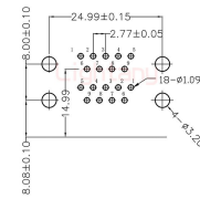
PCB布局 (PCB Layout)
