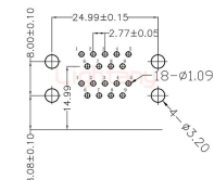
PCB布局 (PCB Layout)
