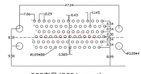
PCB布局 (PCB Layout)
