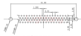
PCB布局 (PCB Layout)
